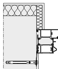
Blokktok Szerelőfüles rögzítés
