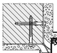
Beépítés tiplis rögzítőfülekkel
