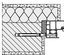
Blokktok Szerelés szerelőnyíláson át
