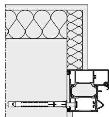
Blokktok Szerelés szerelőnyíláson át
