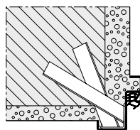
Beépítés horgonyos rögzítőelemmel
