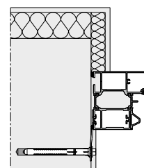
Blokktok nyílásba építéshez (21101 jelű profil)
