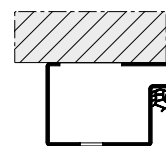
Blokktok falra szereléshez (006 jelű profil) (a pánttal ellentétes oldalra bevizsgálva)
