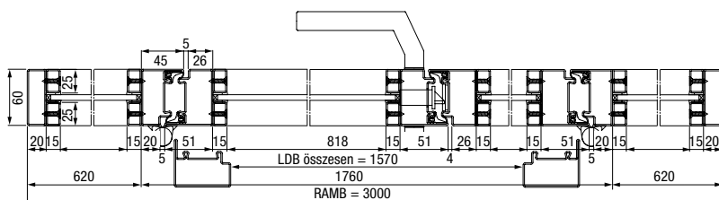
Vízszintes metszet
