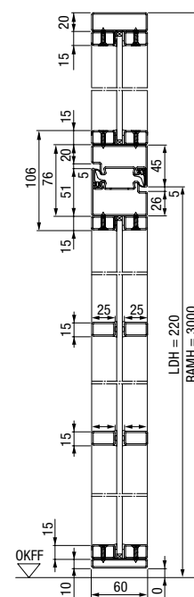
Függőleges metszet
