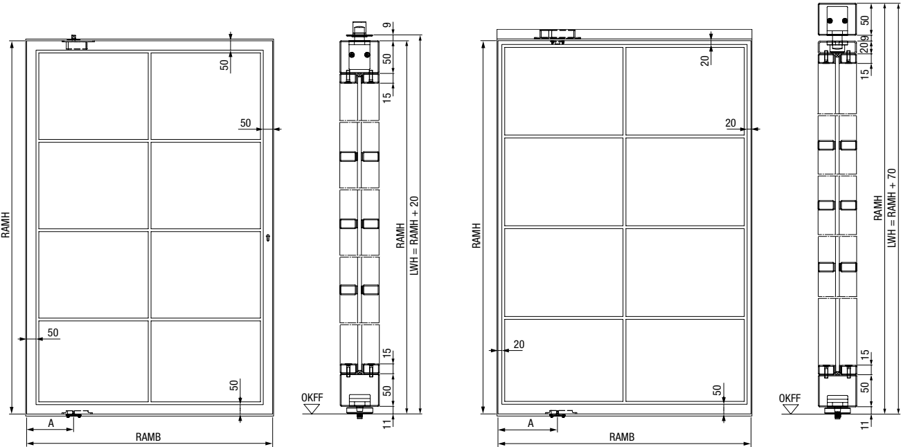
Pivot ajtó alapkivitelben 50 mm széles keretprofillal és 50 mm magas lábazattal, szimmetrikus osztókiosztással
