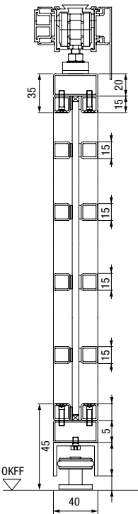
Függőleges metszet
