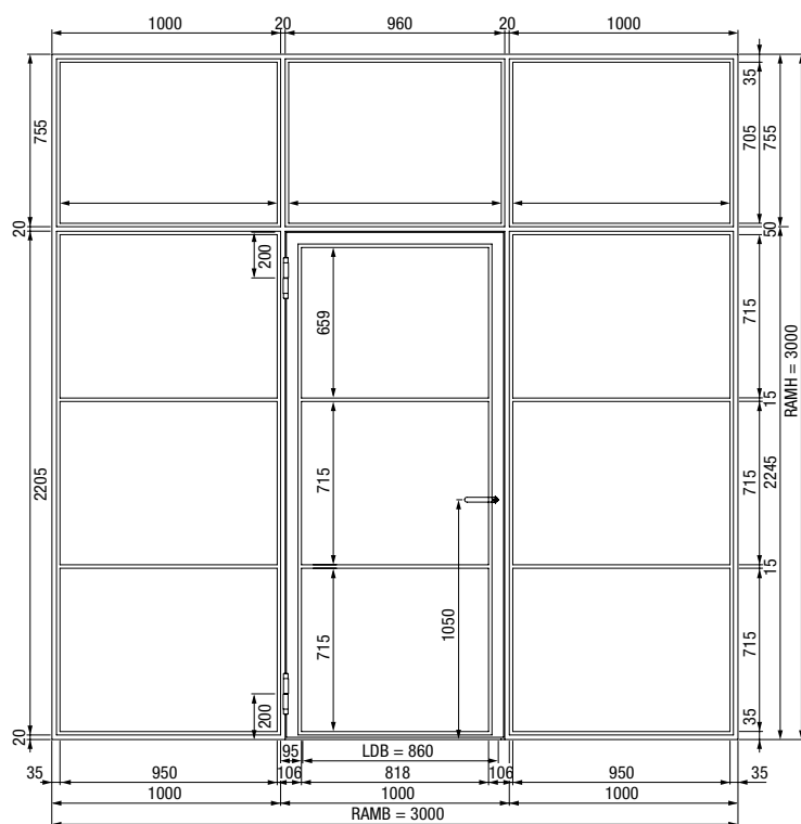
1-szárnyú nyílószárnyas ajtó oldalelemekkel és felülvilágítóval
