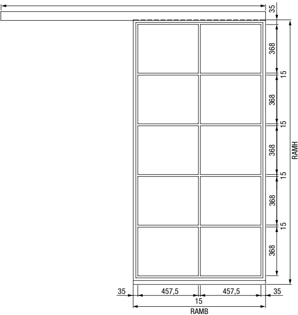
1-szárnyú tolóajtó
