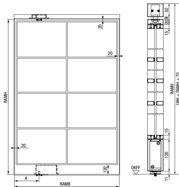
Pivot ajtó 20 mm széles keretprofilal és 120 mm magas lábazattal, szimmetrikus osztókiosztással
