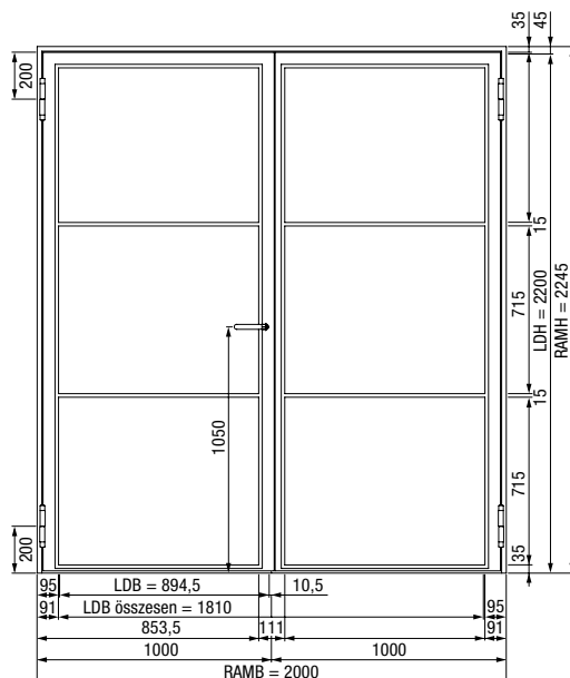
2-szárnyú nyílószárnyas ajtó
