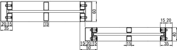
Vízszintes metszet
