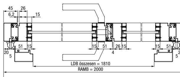
Vízszintes metszet, 2-szárnyú nyílószárnyas ajtó
