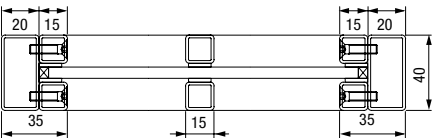
Vízszintes metszet
