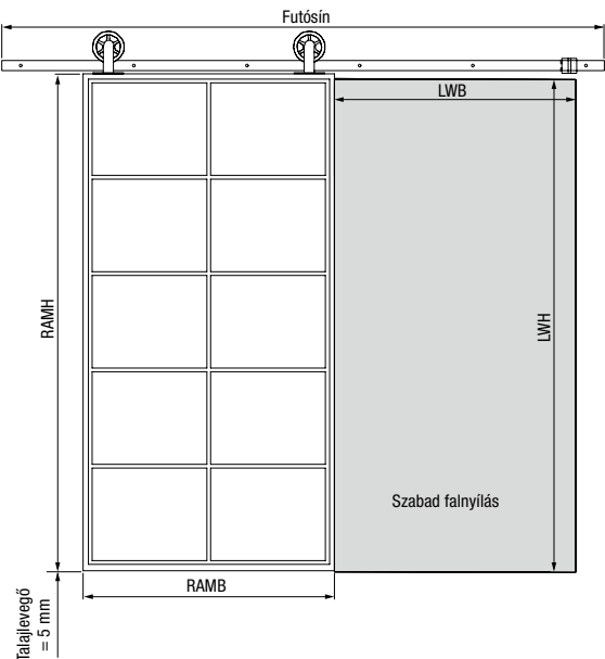
1-szárnyú Retro Loft tolóajtó
