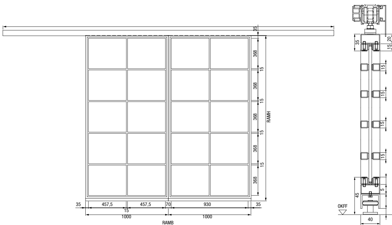
1-szárnyú tolóajtó
