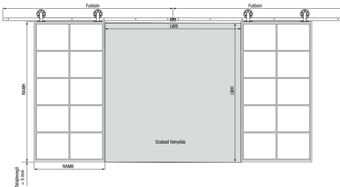
2-szárnyú Retro Loft tolóajtó
