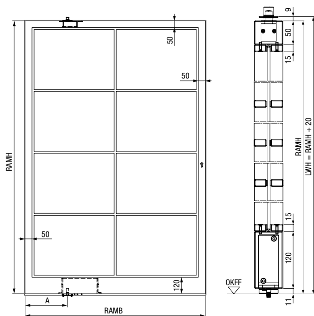
Pivot ajtó 50 mm széles keretprofilal és 120 mm magas lábazattal, szimmetrikus osztókiosztással
