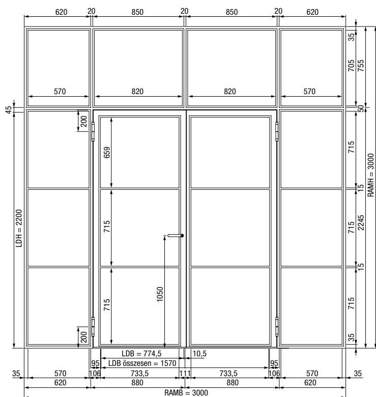
2-szárnyú nyílászárnyas ajtó oldalelemekkel és felülvilágítóval
