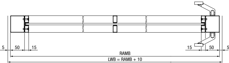
Vízszintes metszet, pivot ajtó alapkivitelben, szimmetrikus osztókiosztással
